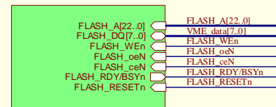
DAB64x_Flash.SchDoc
