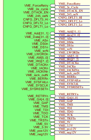
DAB64x_VME_Interface.SchDoc
