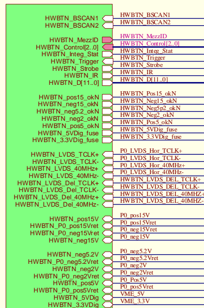
DAB64x_HWBTN.SchDoc
