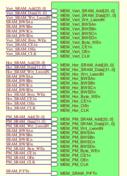
DAB64x_Synch_SRAM.SchDoc
