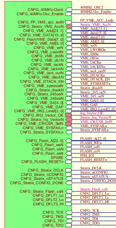
DAB64x_Stratix_Configurator.SCHDOC
