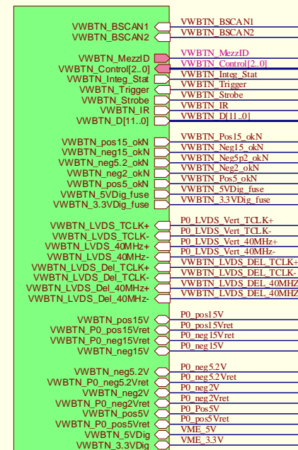
DAB64x_VWBTN.SchDoc
